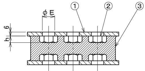
X-X' 断面図
